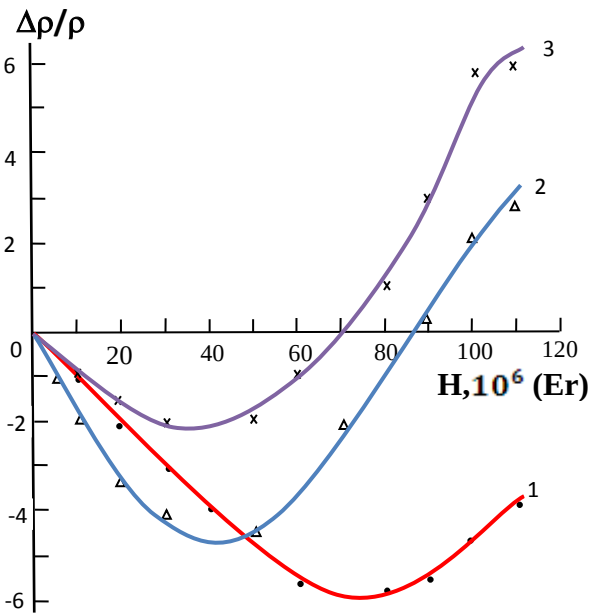
Şəkil 2. (\text{SnSe})_{1-x}(\text{DySe})_x ərintilərinin maqnit müqavimətinin sahə intensivliyindən asılılığı: T=105 K. 1- x=0,005 ; 2- x=0,01 ; 3- x=0,02
