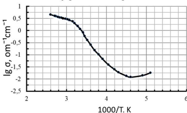
Şəkil1. \text{AgIn}_5\text{S}_8 kristalında elektrik keçiriciliyin temperatur asılılığı
