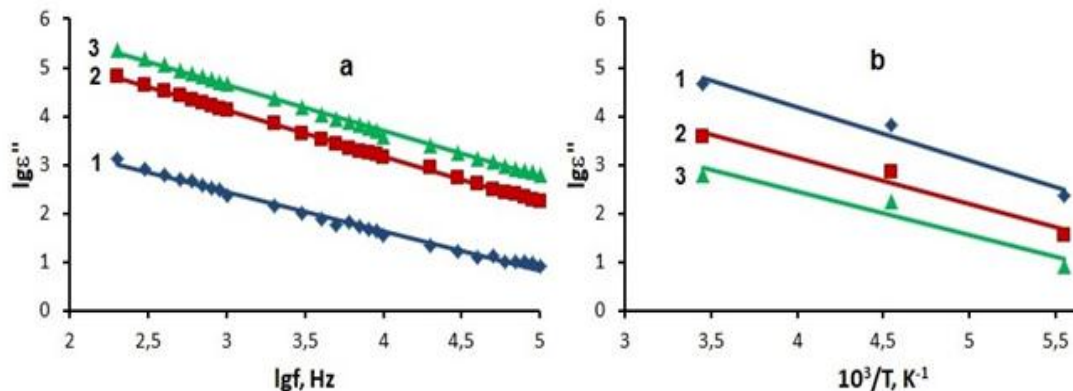
Şəkil 2. \text{MnIn}_2\text{Se}_4 kristalı üçün (a) müxtəlif temperaturlarda \lg \varepsilon'' - \lg f asılılığı ( T, \text{K} : 1–180; 2–220; 3–290); (b) elektrik sahəsinin müxtəlif tezliklərində \lg \varepsilon'' - 10^3/T asılılığı ( f, \text{Hz} : 1– 10^3 ; 2– 10^4 ; 3– 10^5 ).
