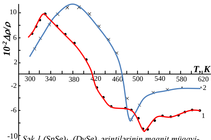
Şəkl. 1. (\text{SnSe})_{1-x}(\text{DySe})_x ərintilərinin maqnit müqavimətinin temperatur asılılığı. 1- x=0,025 ; 2- x=0,04
