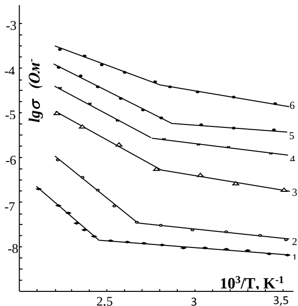
Рис.1. Электропроводности для пленок Ba 0.8 Sr 0.2 TiO 3 при различных частотах: 1-25, 2-10 2 , 3-10 3 , 4-10 4 , 5-10 5 , 6-10 6 Гц
