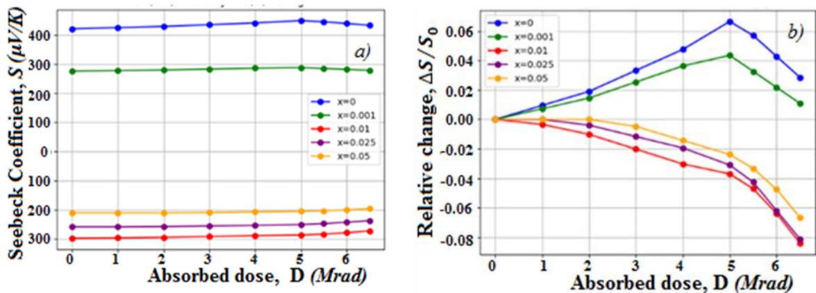
Şəkil 1. Seebeck əmsalının a) və onun nisbi dəyişikliyinə b) udulmuş dozadan asılılığı (Şəkil 1b). n-tip nümunələr üçün isə mənfi qiymətlər alır ( -7 – -8\% -ə qədər). \Delta S/S_0(D) asılılığı qeyri-xəttidir və aşağıdakı kvadratik funksiya ilə yaxşı aproksimasiya olunur:
