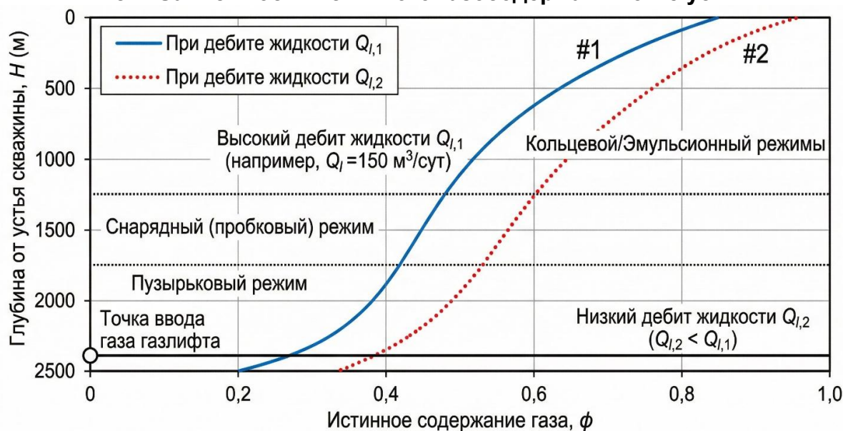
Рис.1. Зависимость истинного газосодержания от глубины
