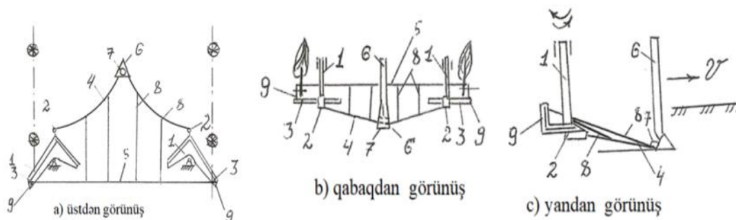
Şəkil 1. 1-dönəbilən pəncə, 2-pəncənin boltu, 3-uzun qanad, 4- elastiki işçi orqan, 5- bərkidici, 6-yumşaldıcı pəncə, 7-diyircək, 8- darayıcı elastiki dartılma, 9- şaquli barmaq.
