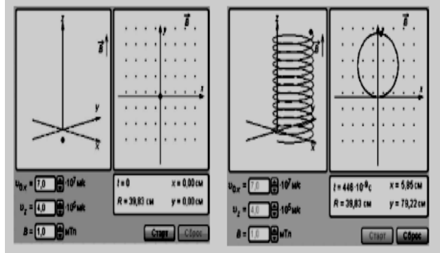
Şəkil . Maqnit sahəsində yüklü zərrəciyin hərəkətini göstərən model
