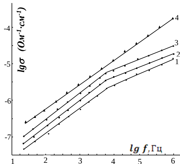
Рис.2. Частотная зависимости проводности пленок \text{Ba}_{0.8}\text{Sr}_{0.2}\text{TiO}_3 : 1-293 К, 2- 373 К, 3-423 К, 4-453К.
