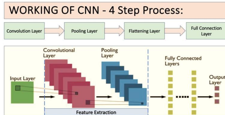
Şəkil 4. Konvolyusiya neyron şəbəkəsi (CNN) əsasında obyekt tanıma prosesinin mərhələli strukturu.
