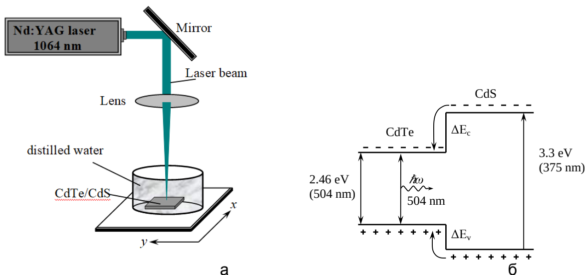
Рис.1. а- Схема экспериментальной установки для абляции наночастиц CdTe/CdS; б- Зонная диаграмма наногетероструктуры CdTe/CdS.
