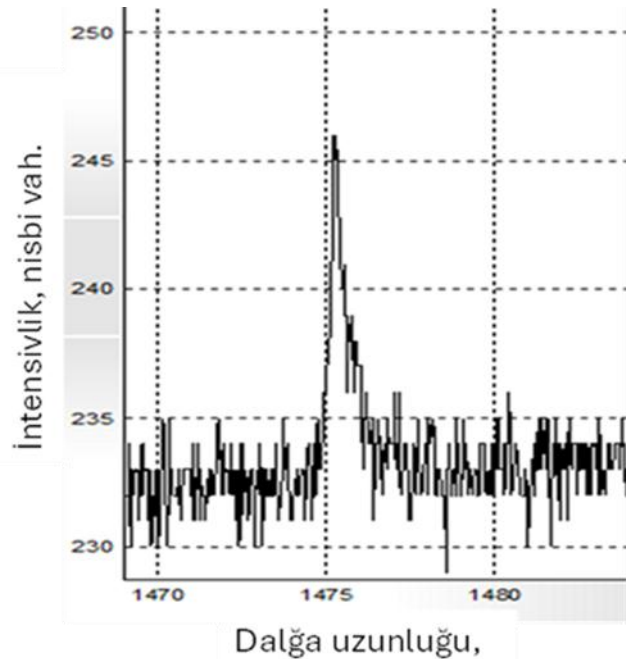
Şəkil 1. AgIn 5 S 8 kristalında fotoluminessensiya spektri.
