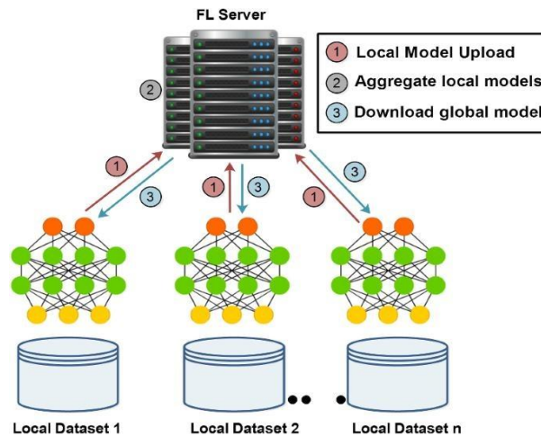
Şəkil 3. Federativ öyrənmə (Federated Learning) arxitekturası
