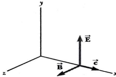
Şəkil 1. \vec{B} , \vec{E} və \vec{c} vektorlarının istiqamətlərinin sxematik təsviri.
