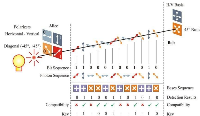
Şəkil 1. BB84 protokolunun işləmə arxitekturası
