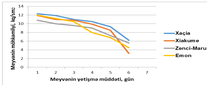
Şək. 1. Yetişmə dərəcəsindən asılı olaraq meyvənin mexaniki möhkəmliyinin dəyişməsi
