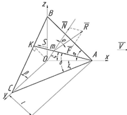
Şəkil 1. Pazın döşəmə materialı ilə təmas sxemi.
