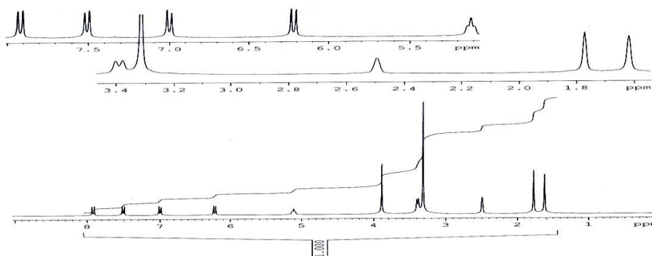
Şək. 2. Ostolun 1 H NMR-spektri.
